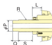
PU203～PU205 (ドロワー接続部)
