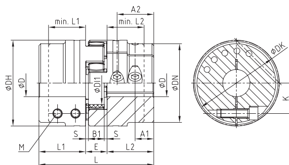
ROTEX® 38 - 90
