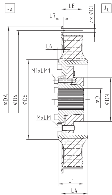
Type AKC
