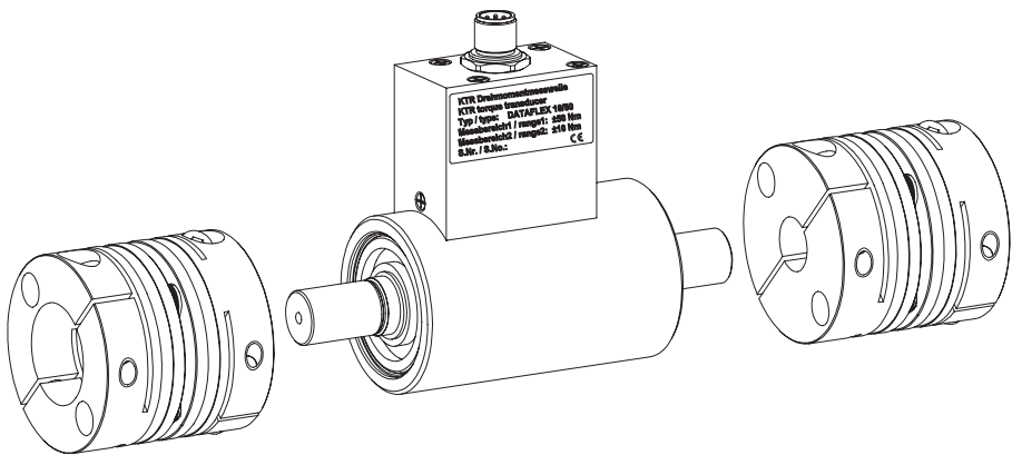
DATAFLEX® 16
