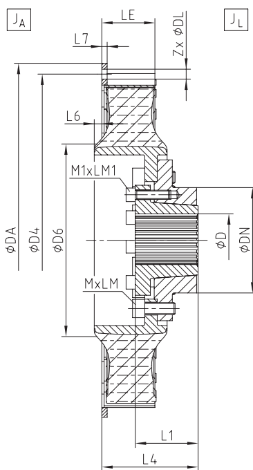
Type ALC
