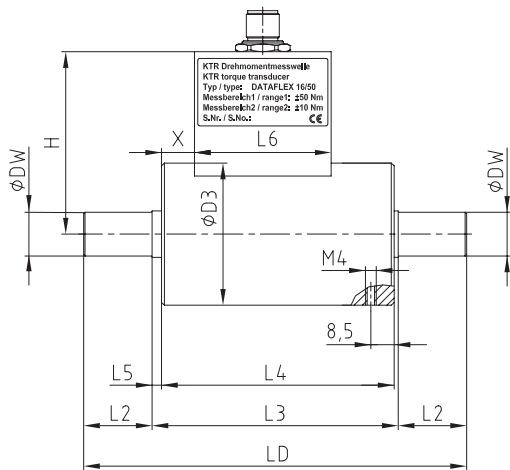
DATAFLEX® 16
