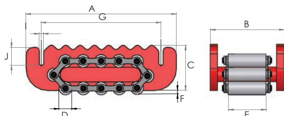
Zeichnungen für Modelle RSN10, RSN15 und RSN30
