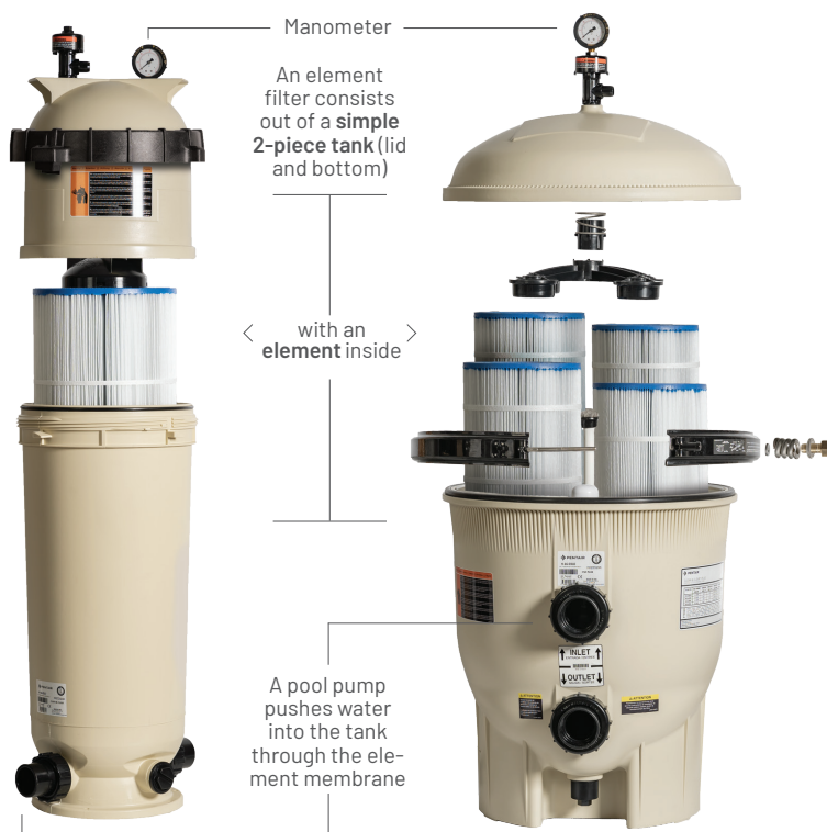
Manometer
