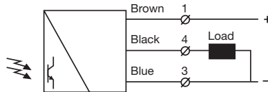
SMR 620x / 630x
